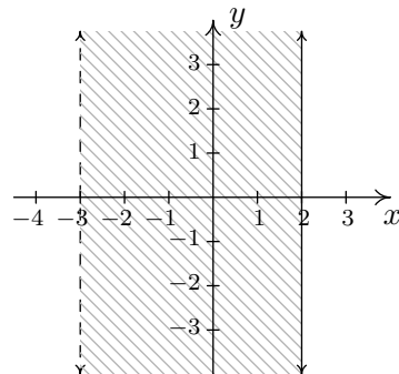
(d) The graph of relation D
